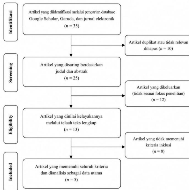
Gambar 1. Langkah-Langkah Seleksi Artikel Berdasarkan PRISMA Sumber: Diadaptasi dari Page et al. (2021)
